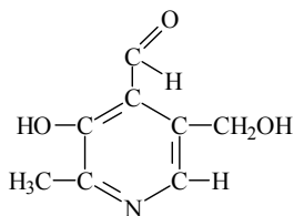
Пиридоксаль
