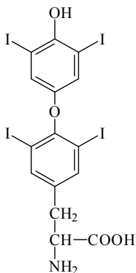
Тироксин
