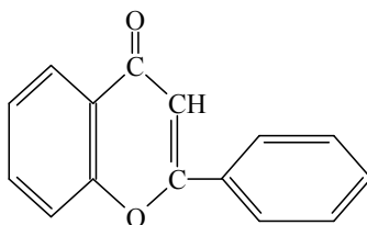
Флавоно
