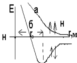
Рисунок 9. Потенциальная энергия системы, состоящей из двух атомов водорода: а - при параллельных спинах электронов; б - при противоположно направленных (антипараллельных) спинах электронов
