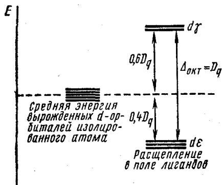
Рисунок 24. Расщепление энергетических уровней d-орбиталей в октаэдрическом поле
